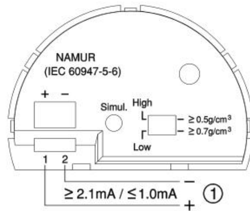
图7 NAMUR 输出方式
