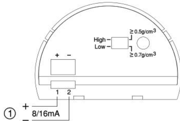
图6 二线制输出方式
