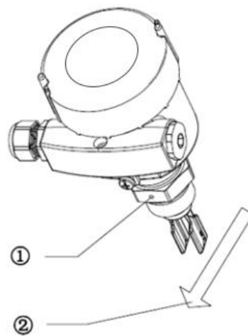
图 2(b) 介质流动方向
