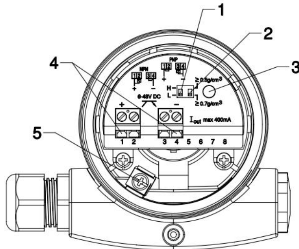
图 14 晶体管(NPN/PNP)输出方式
