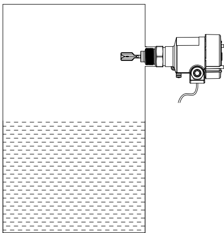
图 2(a) 叉体面垂直安装
