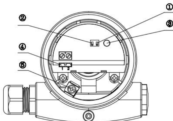
图 12 二线制输出方式
