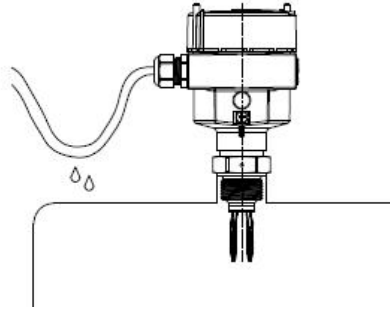
图 4 防潮安装
