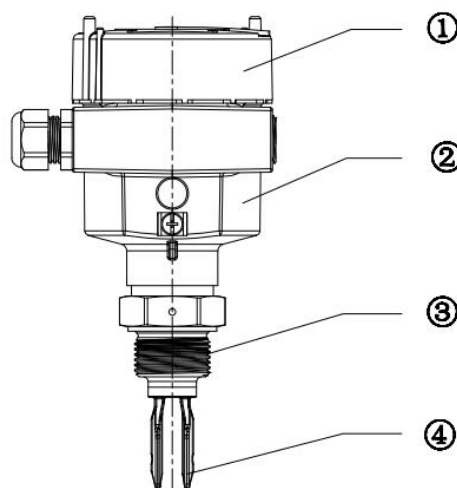
图 1 LTL50 整体结构图
