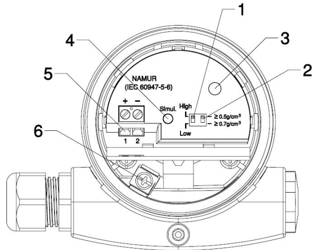
图 13 NAMUR 输出方式
